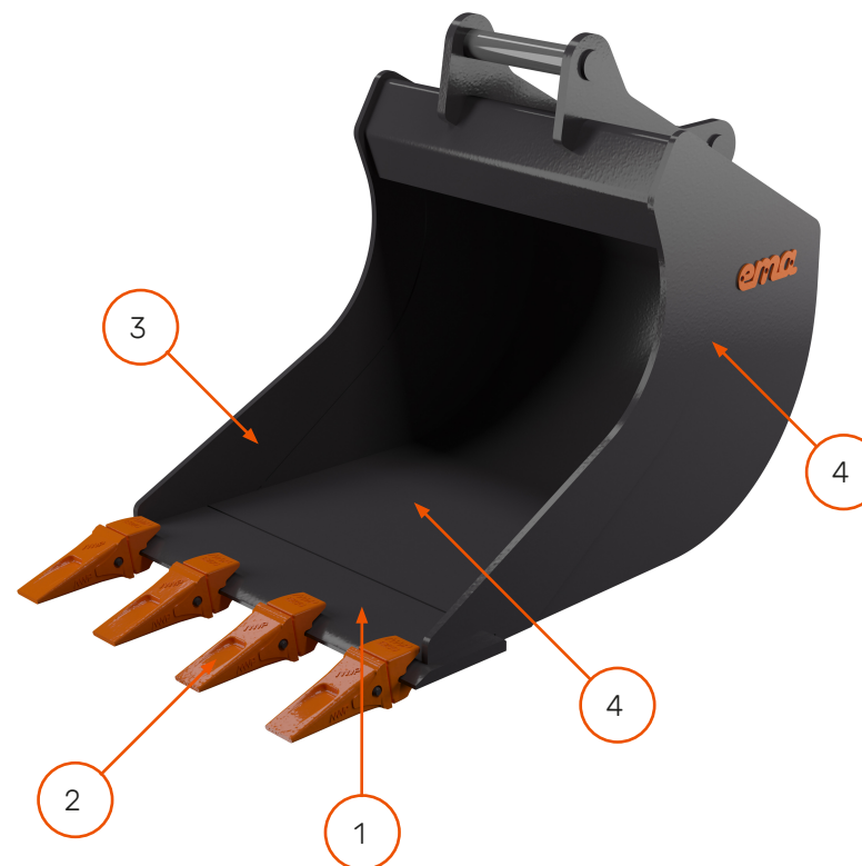
1. Skär 500 Brinell Borox 2. "CAT-tandsystem" 3. Sidoskär/Svep Hardox® 450 4. Sida S355 4. Botten Hardox® 450 VIKTIGT: Bilden visar ett exempel på hur det kan se ut på en viss modell, variationer på andra produktmodeller kan förekomma. Alla produkter är inte godkända enligt Hardox® in My Body. Fråga oss om ni vill veta mer.
