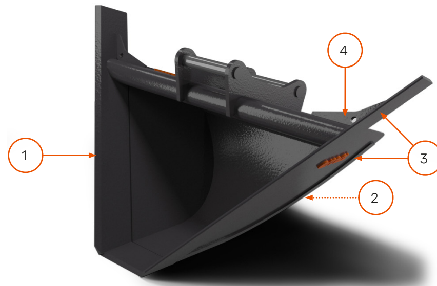
1. Skär Brinell Borox 500 2. Baksida Hardox® 450 3. Kantlist Hardox® 450 4. Förstärkta innersidor VIKTIGT: Bilden visar ett exempel på hur det kan se ut på en viss modell, variationer på andra produktmodeller kan förekomma. Alla produkter är inte godkända enligt Hardox® in My Body. Fråga oss om ni vill veta mer.
